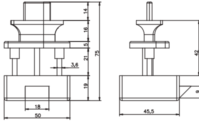
Basmalı Kilit
