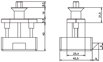
Basmalı Kilit
