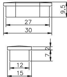
Oval Boru Tapası
